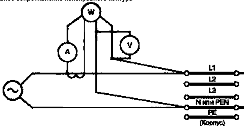
Рисунок DD.1 — Определение активного сопротивления и реактивного сопротивления неисправного контура
