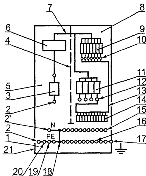
Рисунок Б.4а - Схема расположения аппаратуры в шкафном ВРУ класса II (с изоляционной оболочкой)
