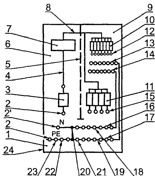
Рисунок Б.3 - Схема расположения аппаратуры в однопанельном ВРУ
