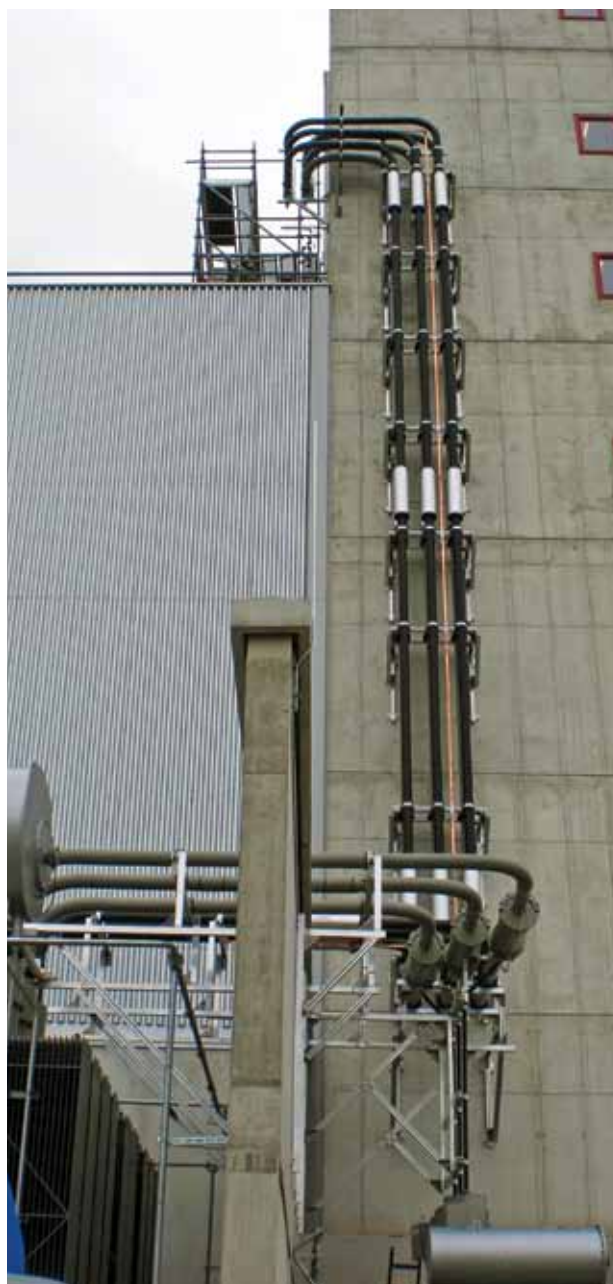
DURESCA 12 кВ 3150 А, 4500 А Соединение генератора с силовым трансформатором (Австрия)
