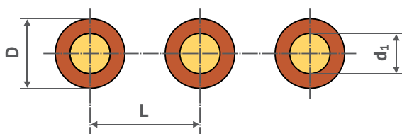
Проводник круглого сечения
