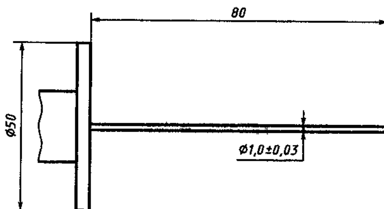
Рисунок 2 - Испытательный щуп
