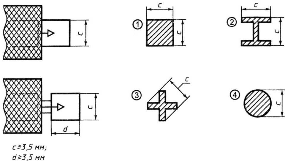
Рисунок 3 - Измеряемые места типичных контактов адаптеров класса III
