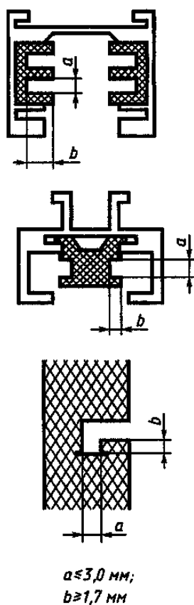
Рисунок 4 - Измеряемые места типичных секций шинопроводов класса I
